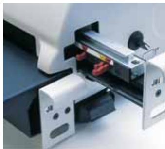
Schnelle und einfache Auswechslung des Stanzwerkzeugs
